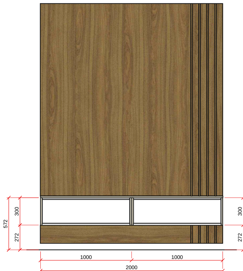
VISTA A - ESC. 1:25
